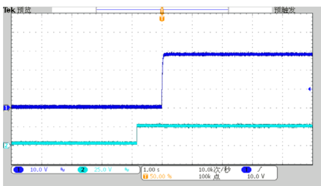
图 (5) 电源开机波形图
