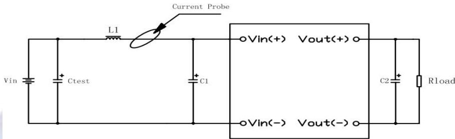
图(15)输入反射纹波电流测试示意图
