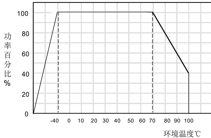
温度/功率降额曲线
